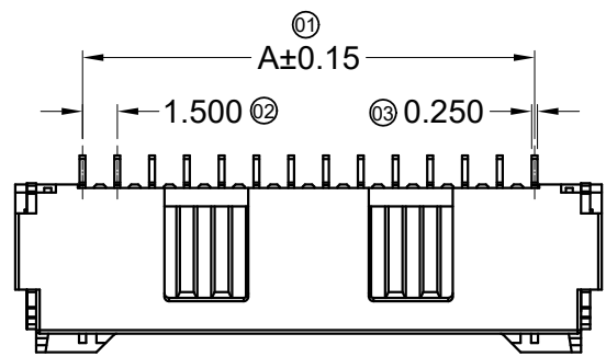
06P-15P Double Hole Scale 1:1
