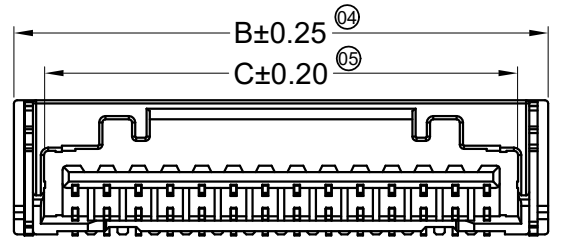
06P-15P Double Hole Scale 1:1
